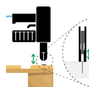
clouer avec un cloueur pneumatique
